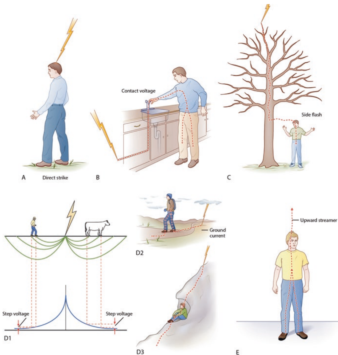
Figura 6.19: Possibili fulminazioni: fulminazione diretta (direct strike - A), scarica per contatto (contact voltage - B), scarica di rimbalzo (side flash - C), tensione di passo (step voltage - D1), corrente di terra (ground current - D2 e D3) e canale ionizzato ascendente (upward streamer - E) [M.A. Cooper e R. L. Holle].
