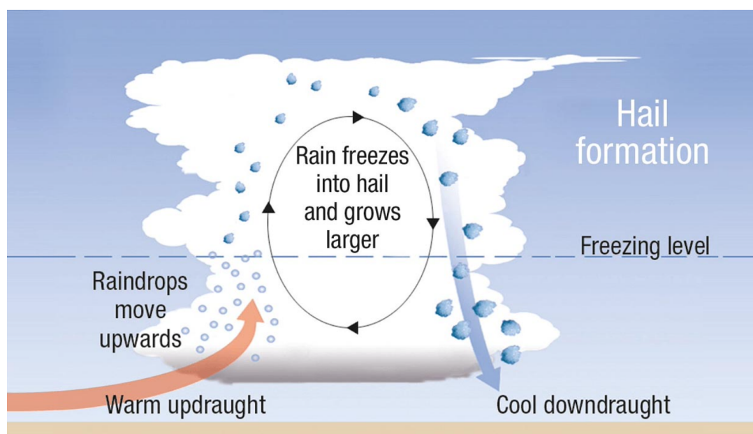
Figura 6.7: Formazione di grandine in un cumulonembo [Severe Weather Europe].
