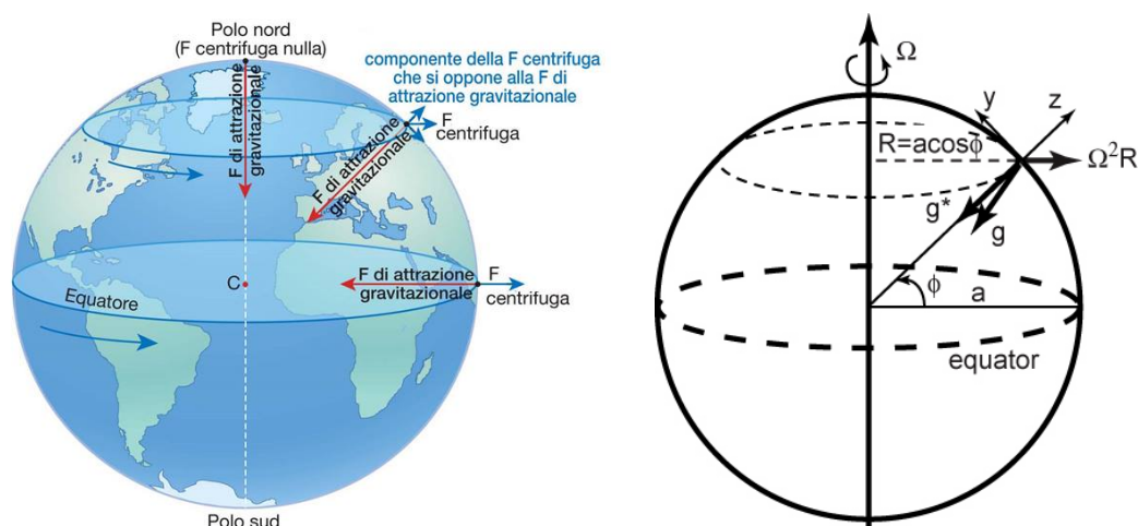
Figura 7.1: A sinistra: in ogni punto della Terra, tranne che ai poli, la componente verticale della forza centrifuga riduce la forza di attrazione Newtoniana [FED Channel]. A destra: schema di valutazione quantitativa della accelerazione gravitazionale apparente g come somma vettoriale di accelerazione gravitazionale newtoniana g^* e accelerazione centrifuga a_{cen} = \Omega^2 R [University of Colorado Boulder].
