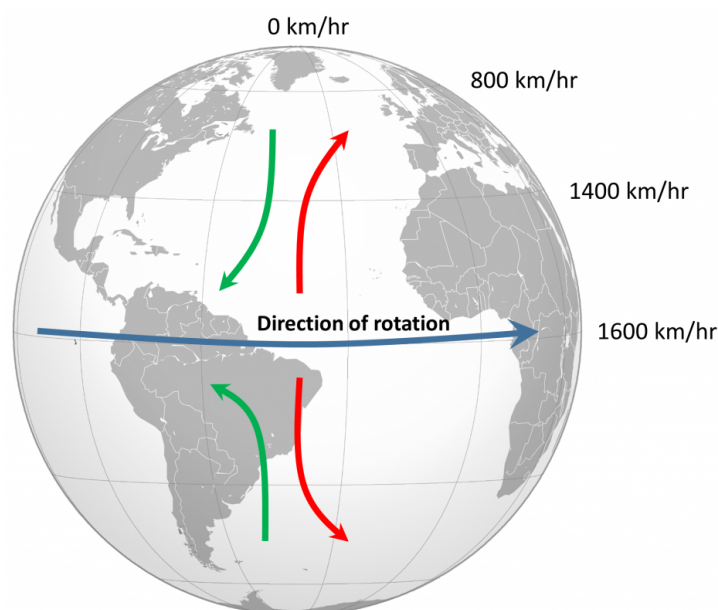
Figura 3.6: Spostamenti lungo i meridiani. In entrambi gli emisferi le masse che si spostano dalle vicinanze dell'equatore verso i poli (freccie rosse) vanno in regioni caratterizzate da velocità periferiche minori e appaiono deviate verso est, mentre le masse che si spostano dalle vicinanze dei poli verso l'equatore (freccie verdi) vanno in regioni caratterizzate da velocità periferiche maggiori e appaiono deviate verso ovest. L'unica differenza è che, rispetto alla direzione di spostamento, le deviazioni sono verso destra nell'emisfero settentrionale e verso sinistra nell'emisfero meridionale [P. Webb].
