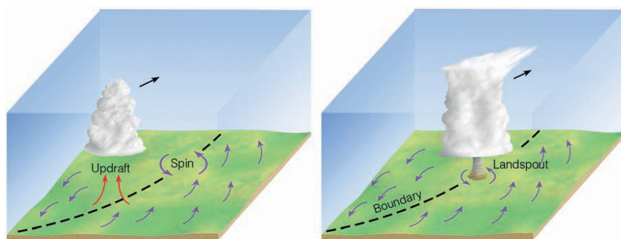
Figura 6.12: Formazione della nube a imbuto in un tornado “non da supercella”. Un cumulo congesto si avvicina ad una perturbazione ciclonica al suolo (a sinistra) e, successivamente, passandole sopra (a destra), la aspira con la sua corrente ascendente [C. D. Ahrens e R. Henson].
