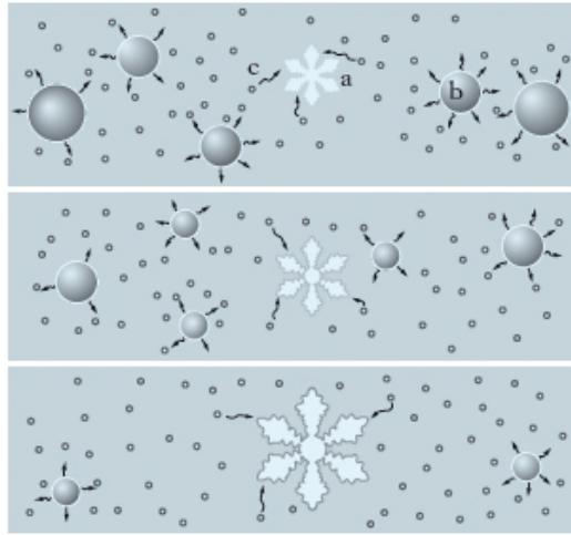
Figura 2.14: Meccanismo di Bergeron, ovvero crescita per condensazione del vapore su un cristallo di ghiaccio a spese dell'evaporazione delle gocce d'acqua soprafusa che lo circondano [Treccani].
