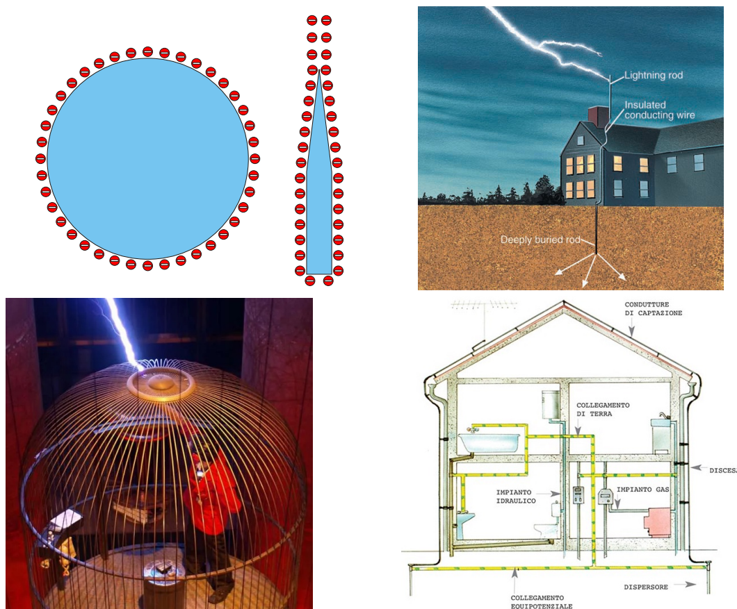
Figura 6.18: Protezione dai fulmini. In alto: a sinistra effetto punta [Wikipedia] e a destra sfruttamento di tale effetto in un impianto parafulmine [C. D. Ahrens e R. Henson]. In basso: a sinistra il principio di funzionamento della Gabbia di Faraday [Wikipedia] e a destra il suo utilizzo negli impianti di protezione degli edifici [Creative Commons].
