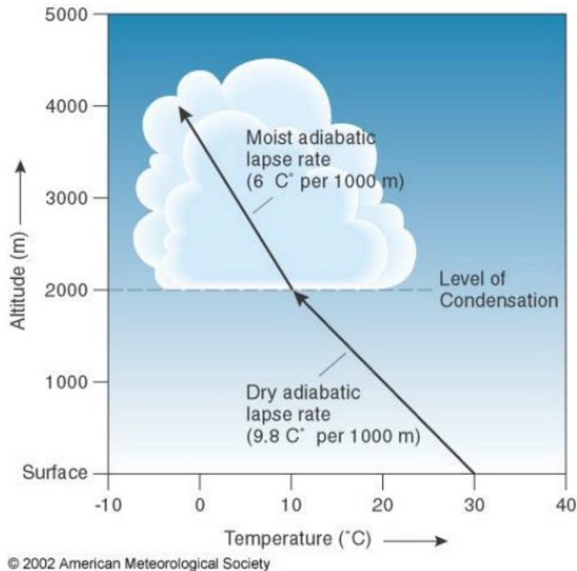
Figura 2.10: Schematizzazione del raffreddamento adiabatico di una massa d'aria che ha luogo “a secco” fino alla quota della temperatura di saturazione e “ad umido” oltre tale quota [American Meteorological Society].
