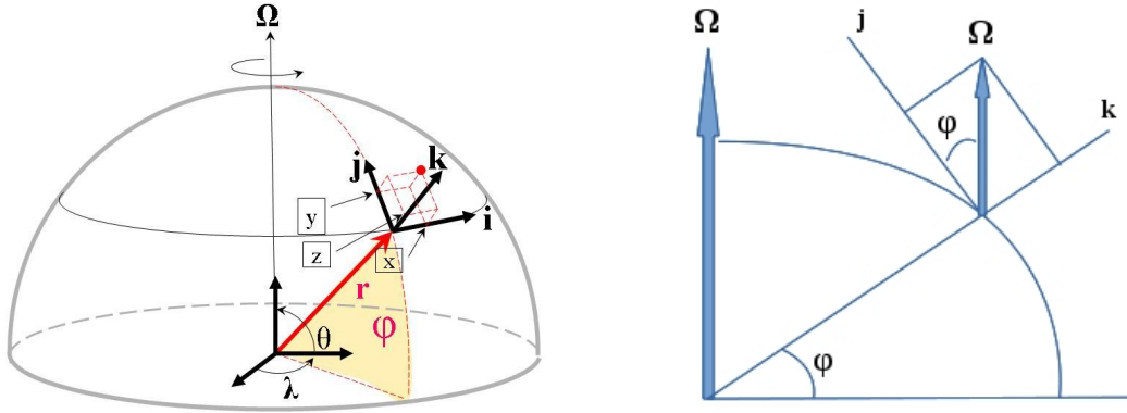
Figura 7.3: A sinistra: sistema di coordinate cartesiane locali, con versori \mathbf{i}, \mathbf{j}, \mathbf{k} , utilizzato per il calcolo delle componenti delle accelerazioni apparenti [Persson]. A destra: sezione meridiana della Terra e calcolo delle componenti locali del vettore velocità angolare \Omega [Centro Meteo].
