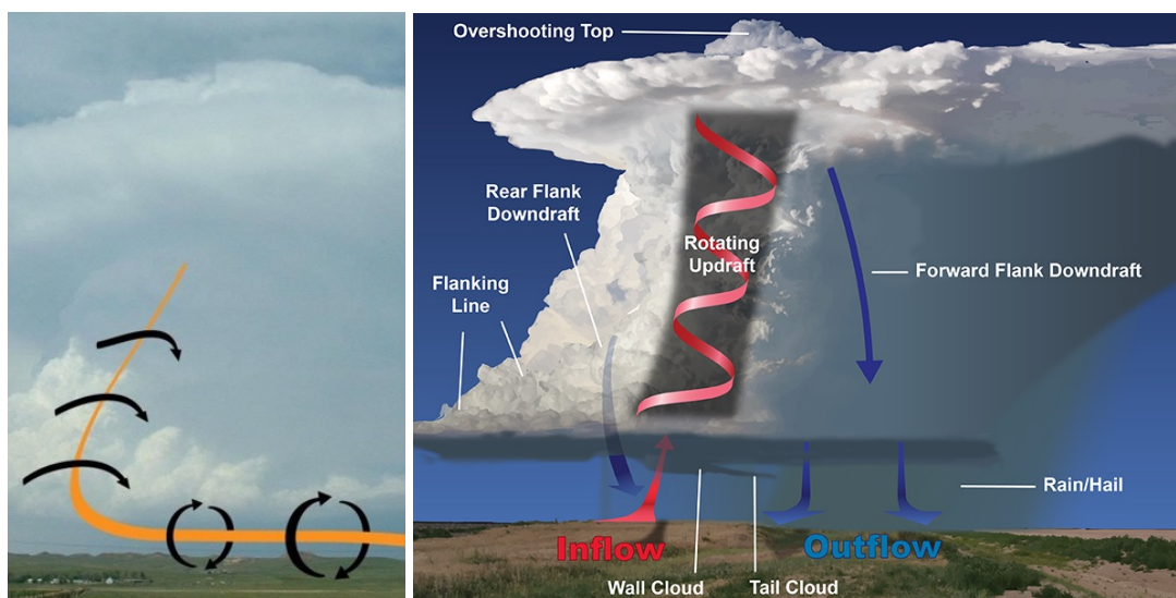
Figura 6.5: Temporali a supercella. A sinistra: genesi del mesociclone che caratterizza le supercelle [Wikipedia]. A destra: struttura finale di una supercella classica [NWS].
