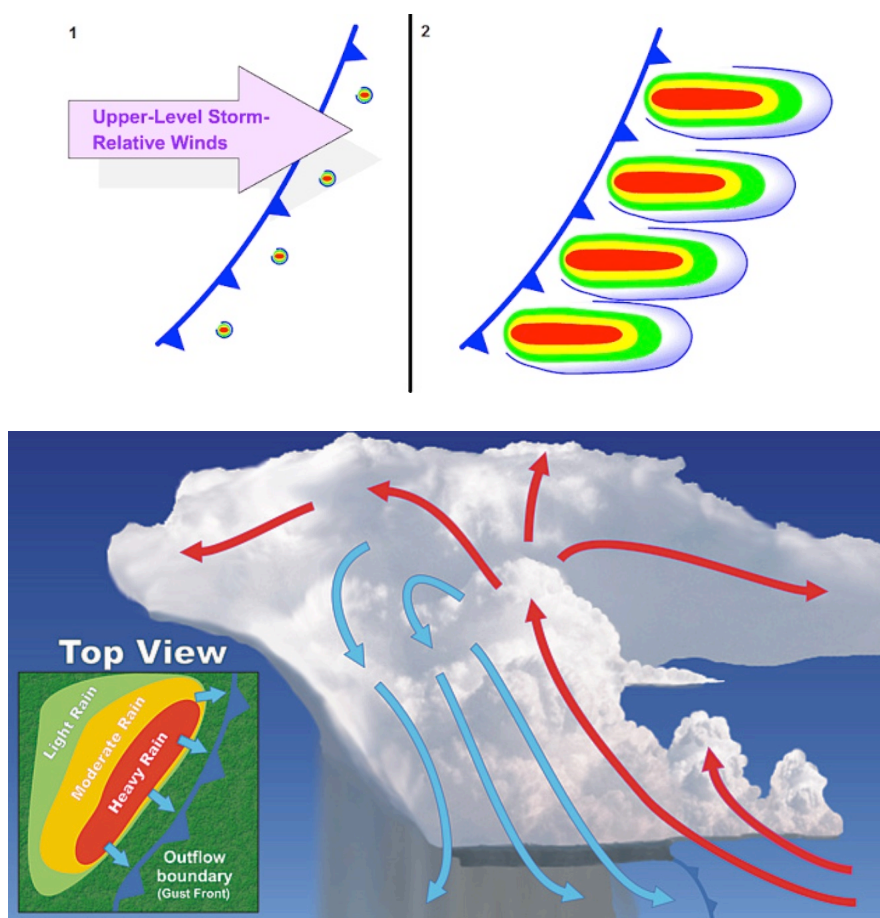
Figura 6.3: Sopra, schema di formazione di una linea di celle (squall line) [Penn State University] e sotto, sezione trasversale della linea con, nell'inserito piccolo, vista in pianta dall'alto della linea in movimento [NOAA].
