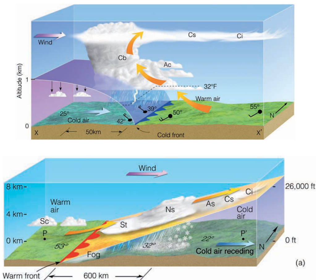
Figura 5.6: In alto: vista tridimensionale di un fronte freddo. In basso: vista tridimensionale di un fronte caldo. Le temperature sono misurate in gradi Fahrenheit (°F) dove 32^{\circ}\text{F} = 0^{\circ}\text{C} e 1^{\circ}\text{F} = 5/9^{\circ}\text{C} [C.D. Ahrens e R. Henson].
