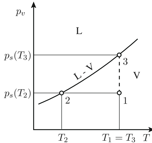
Figura 2.4: Trasformazioni del vapore d'acqua nell'aria a pressione costante \overline{12} ed a temperatura costante \overline{13} , rappresentate nel diagramma (p, T) .
