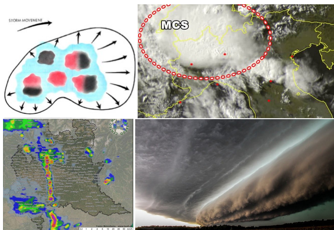
Figura 6.4: Sistema convettivo a mesoscala. Riga in alto: numerosi grappoli di celle che incidono sulla stessa area, con a sinistra schema funzionale del sistema [NWGG] e a destra foto satellitare [Public Domain]. Riga in basso: più linee di celle ravvicinate tra loro in direzione ortogonale al moto, con a sinistra foto satellitare di un temporale sulla Lombardia [Centro Meteo Lombardo] e a destra nube a mensola che molto spesso accompagna temporali di questo tipo [Meteo Regione Lazio].
