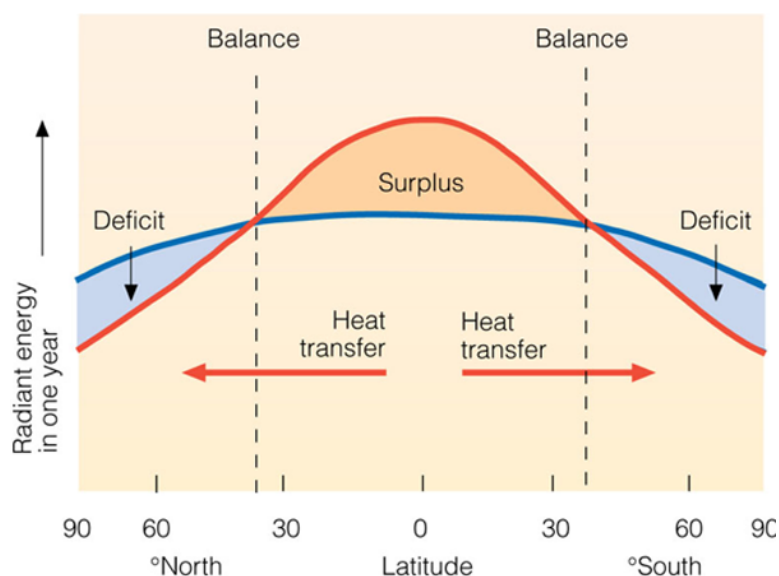
Figura 3.1: Bilanciamento tra radiazione solare annuale assorbita (rosso) e radiazione infrarossa annuale emessa (blu) attraverso i flussi termici convettivi legati alla circolazione atmosferica generale (87% circa) e alle correnti oceaniche su scala planetaria (13% circa) [Nasa].
