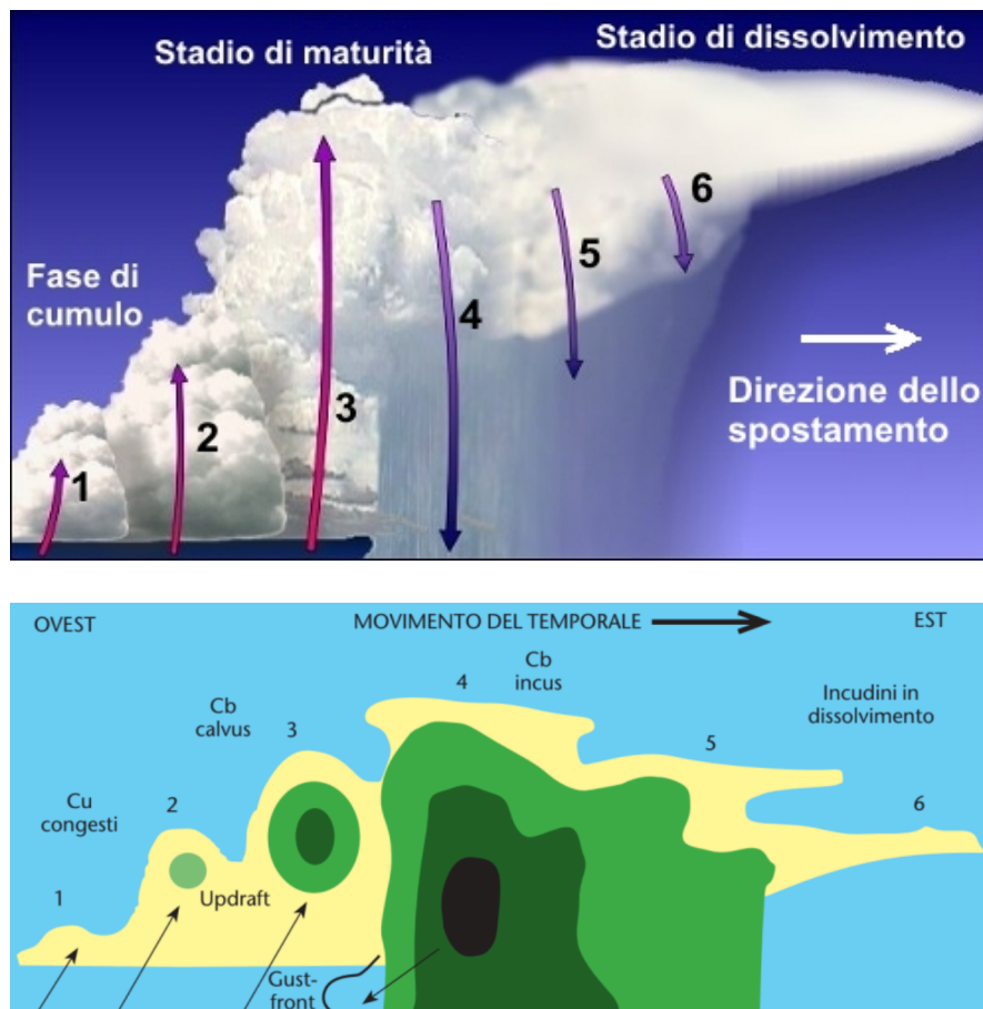
Figura 6.2: Sezione trasversale di un grappolo di celle in movimento sopra [NOAA, modificata] e schema di formazione del grappolo sotto [A. Gobbi, A. Griffa e P. Rinaldi].
