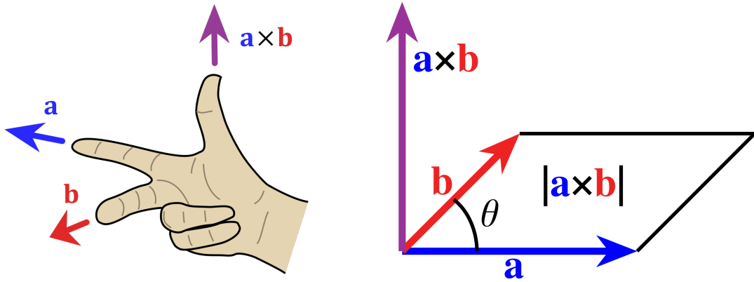
Figura 7.4: A sinistra: la relazione spaziale tra i vettori \mathbf{a} , \mathbf{b} e il prodotto vettoriale \mathbf{a} \times \mathbf{b} è data dalla regola della mano destra. A destra: l'area del parallelogramma individuato dai vettori \mathbf{a} e \mathbf{b} è proporzionale al valore assoluto del loro prodotto vettoriale [Wikipedia].
