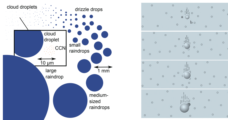
Figura 2.13: Dimensioni in scala di gocce di pioggia, goccioline e nuclei di condensazione, a sinistra [J. Shonk]. Coalescenza, ovvero aggregazione per urto delle gocce piccole da parte delle gocce grandi, a destra [Treccani].
