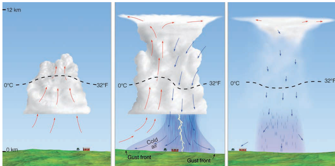
Figura 6.1: Schematizzazione del ciclo di vita di un cumulonembo nel contesto di un temporale di calore estivo a monocella quasi stazionario: sviluppo (a sinistra); maturazione (al centro) e dissolvimento (a destra) [C.D. Ahrens e R. Henson].
