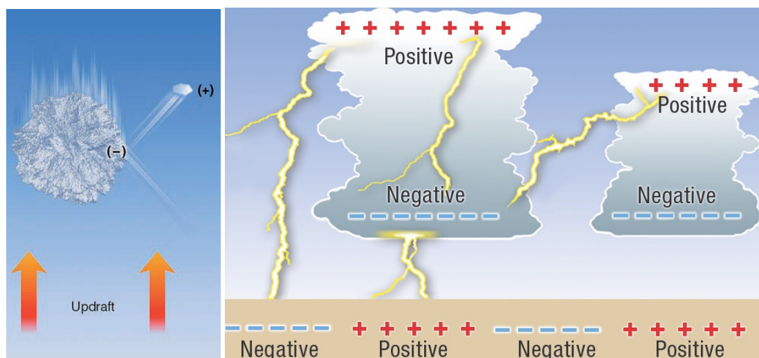
Figura 6.15: Processi di carica nelle nubi. A sinistra: collisione con trasferimento di un elettrone tra una microparticella di ghiaccio che sale e un chicco di gragnola che scende [C. D. Ahrens e R. Henson]. A destra: principali tipologie di fulmini che si possono avere nella situazione finale risultante: intranube, nube-nube, parte bassa negativa di una nube-suolo positivo, parte alta positiva di una nube e suolo negativo [Australian Government].
