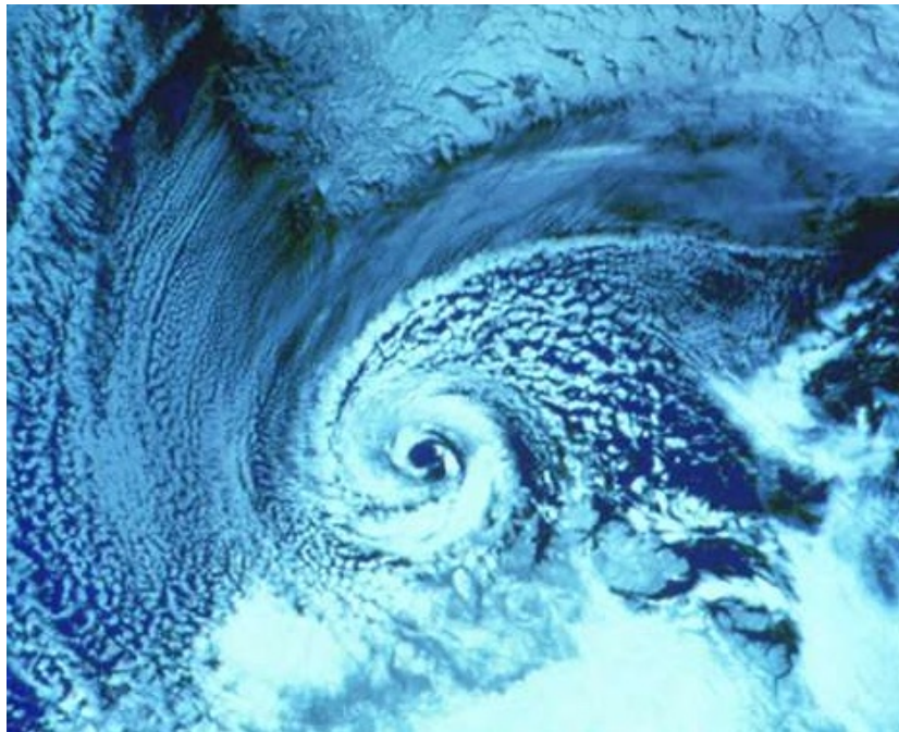
Figura 5.18: Tempesta artica sul Mare di Barents il 27 February 1987 [Wikipedia].
