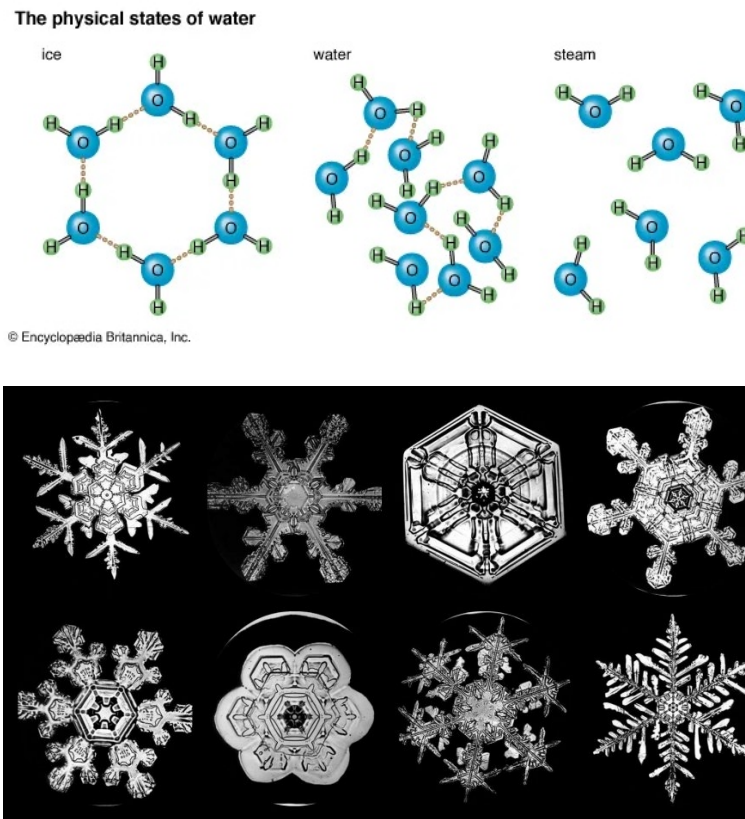
Figura 2.15: Stati fisici dell'acqua, sopra [Enciclopedia Britannica] e fiocchi di neve, sotto [W. Bentley].
