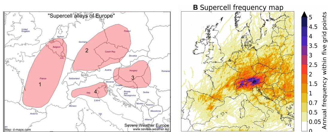
Figura 6.8: Attuali “Supercell Alleys” europee a sinistra [ Severe Weather Europe ] e futura unica “Supercell Alley” a destra dopo l’eventuale probabile aumento futuro di 3 °C nella temperatura media globale europea [ M. Feldmann e altri ].
