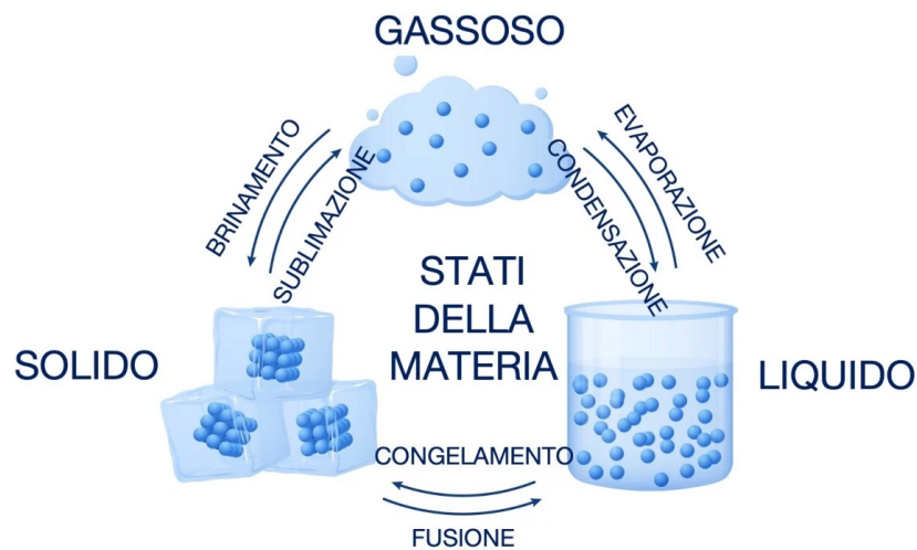
Figura 2.11: Nomenclatura tecnica italiana adottata per i cambiamenti di fase [WAU].
