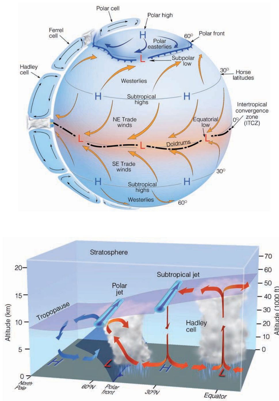
Figura 3.10: Modello a tre celle della circolazione generale dell'atmosfera. In alto: aree di alta e bassa pressione e venti dominanti al suolo e, in basso: sezione meridiana che illustra la formazione dei venti dominanti in quota [C.D. Ahrens e R. Henson].
