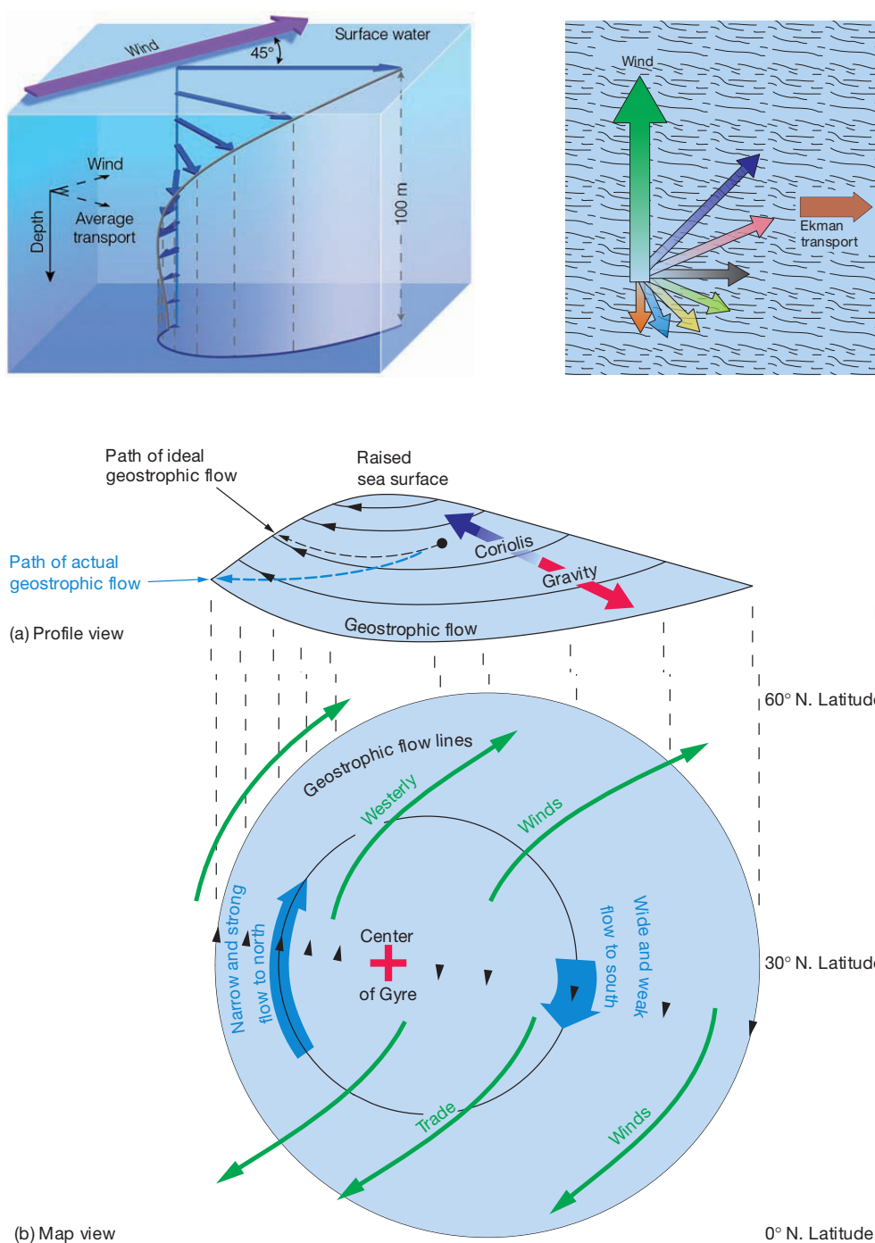
Figura 4.5: Trasporto di Ekman nell'emisfero nord (con ovest a sinistra ed est a destra della figura). In alto: vista prospettica a sinistra [C.D. Ahrens e R. Henson] e vista in pianta a destra [A. Trujillo e H. Thurman]. In basso: correnti geostrofiche viste in profilo sopra e intensificazione occidentale delle correnti geostrofiche vista in pianta sotto [A. Trujillo e H. Thurman].
