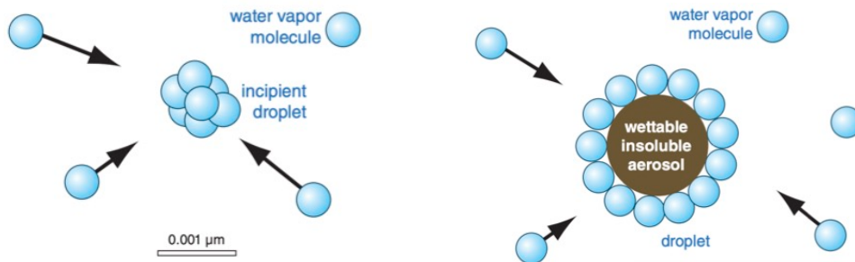
Figura 2.12: Nucleazione omogenea a sinistra ed eterogenea a destra [R. Stull].
